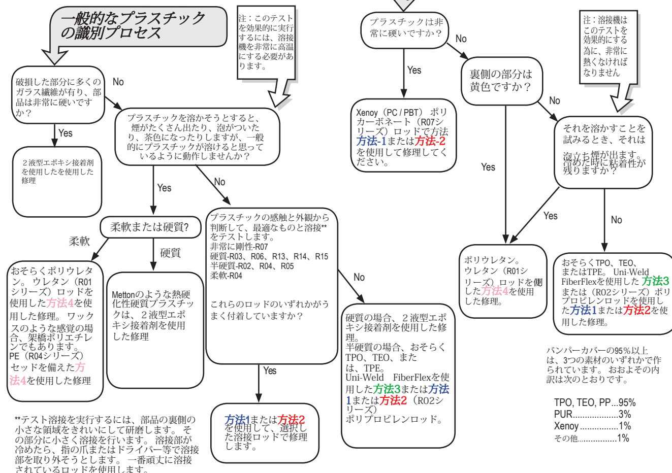
プラスチック修理のクイック照合チャート
